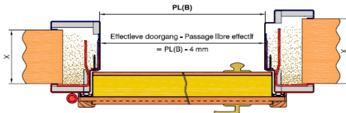
Horizontale Doorsnede - Coupe Horizontale
